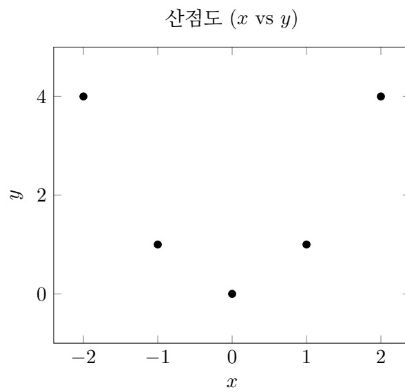
Figure 4: 2.10(a) 산점도: 포물선 형태, 이차함수 관계
