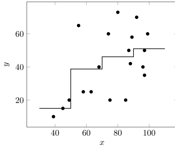
Figure 3: 2.9(a) 과제성적과 시험성적의 산점도 및 회귀도
