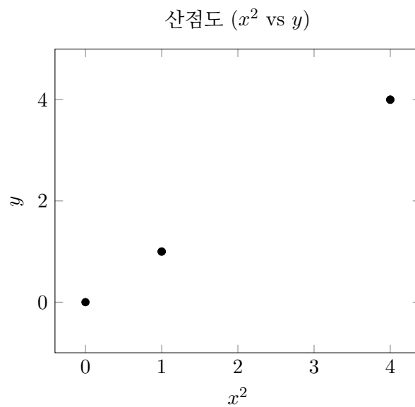
Figure 5: 2.10(c) x^2 와 y 의 산점도: 선형 상관관계
