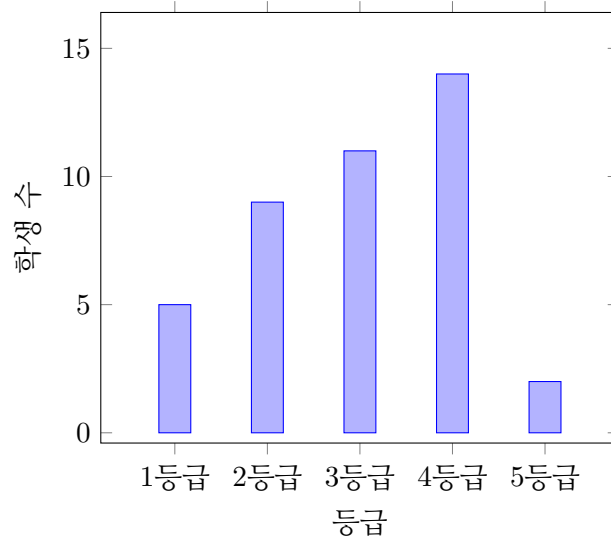
Figure 1: 2.6(c) 성적 등급별 학생 수 막대그래프
