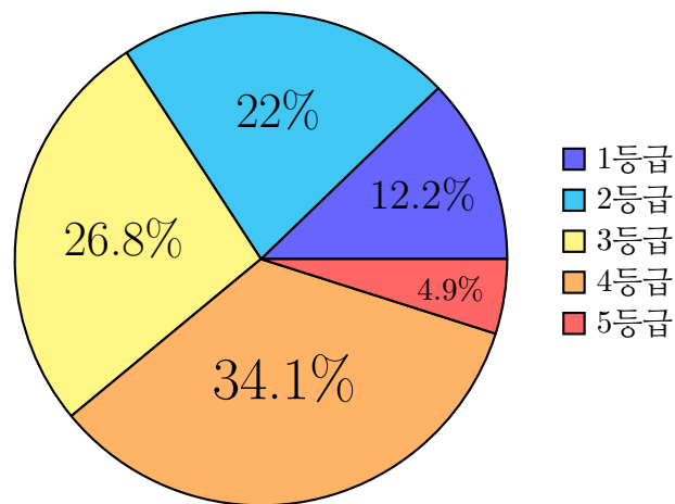
Figure 2: 2.6(c) 성적 등급별 학생 비율 원형그래프 (반올림)
