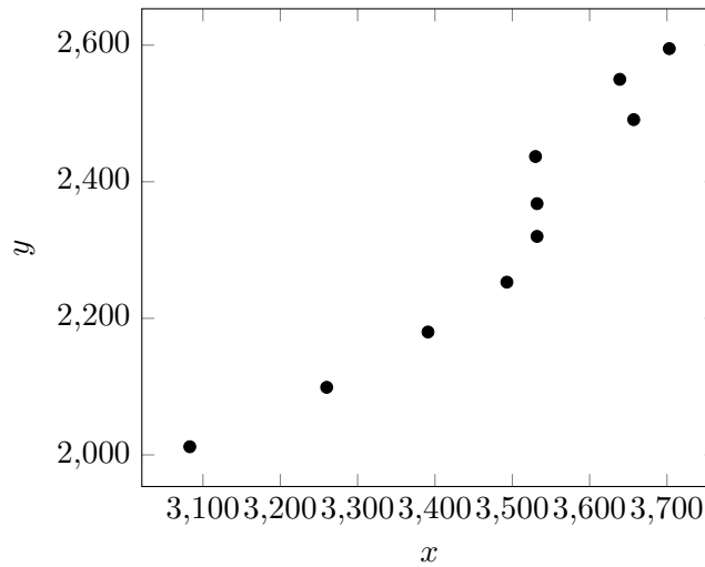
Figure 6: 국민총소득과 자동차 등록대수의 산점도
