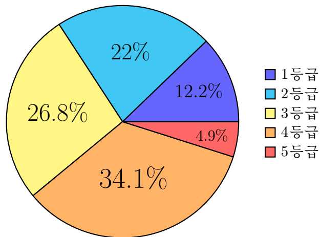
Figure 2: 성적 등급별 학생 비율 원형그래프 (반올림)
