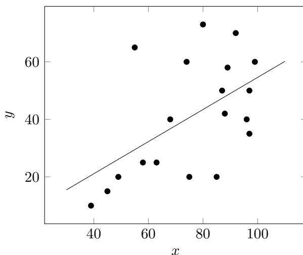
Figure 3: 과제성적과 시험성적의 산점도 및 회귀직선 \hat{y} = -1.2618 + 0.5585x
