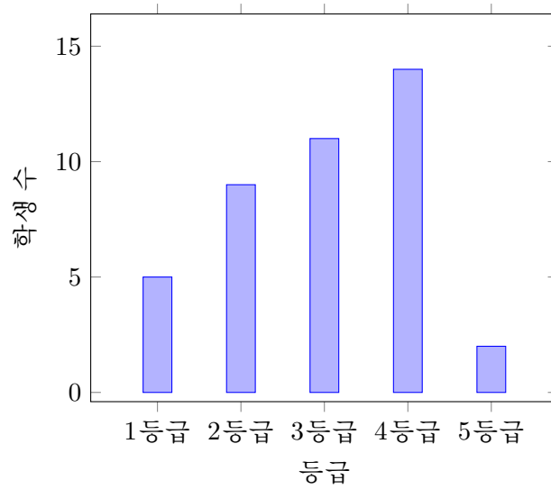
Figure 1: 성적 등급별 학생 수 막대그래프
